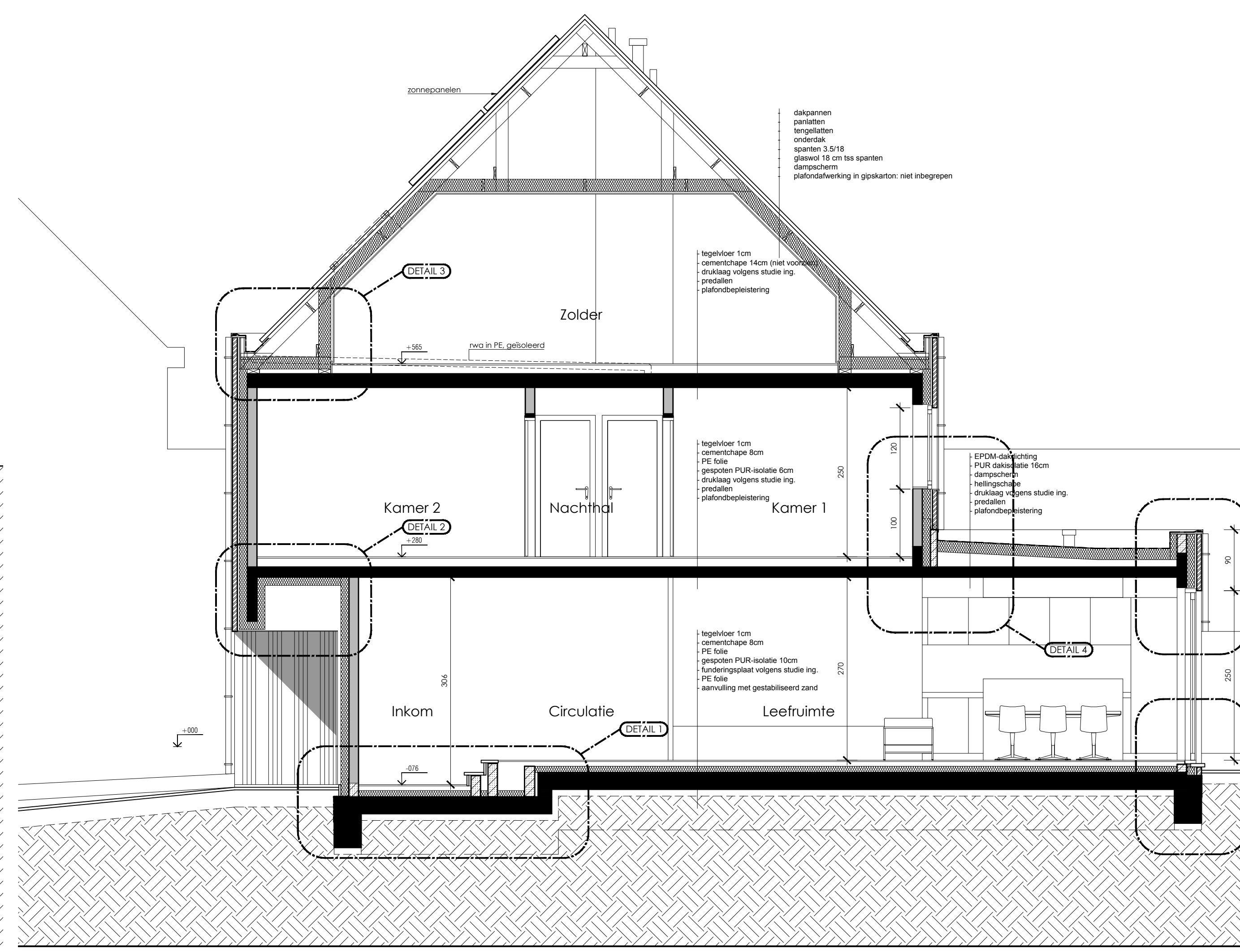
DOORSNEDE AB
