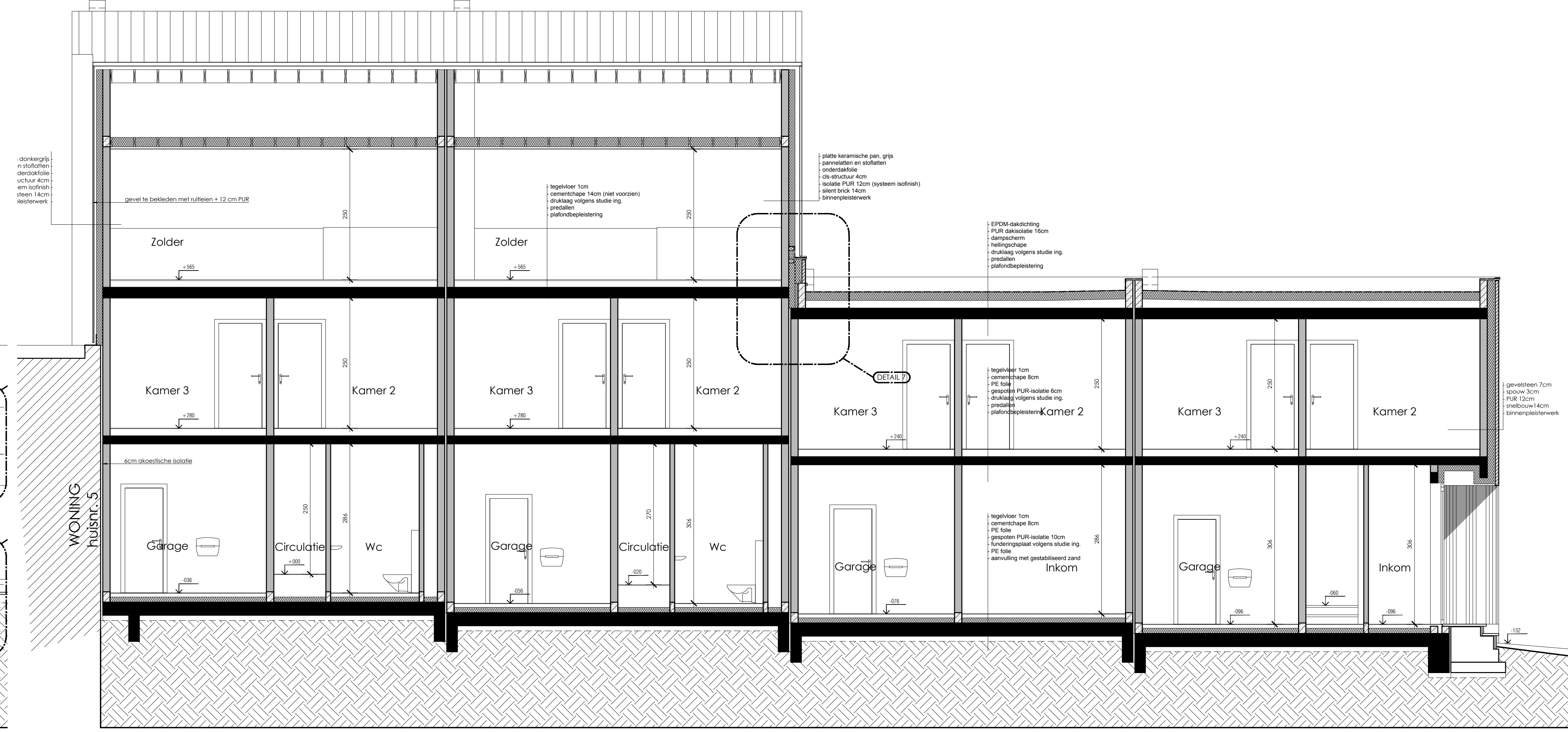
DOORSNEDE CD
